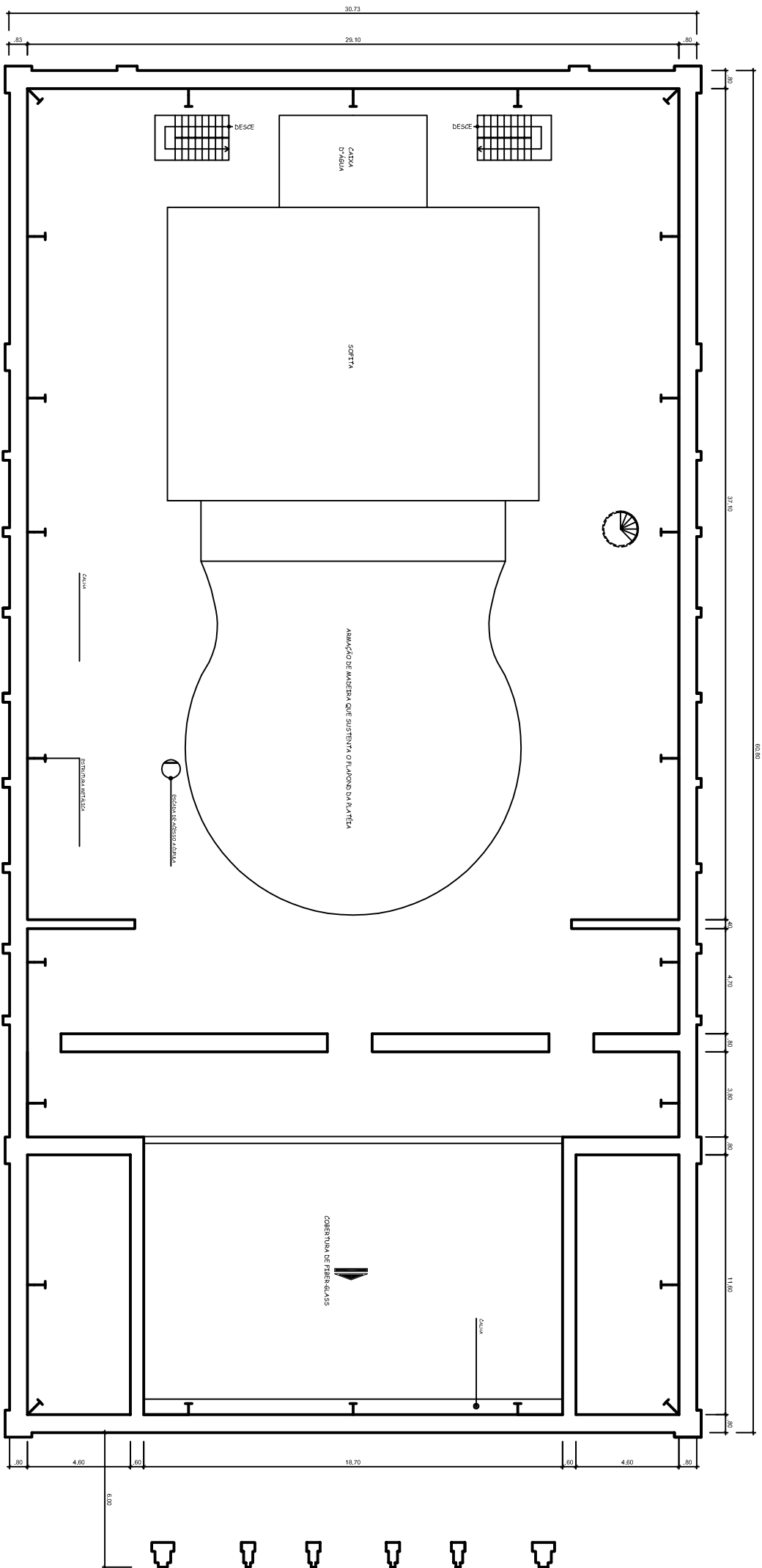
PLANTA BAIXA DA URDIDURA ESCALA: 1/100
